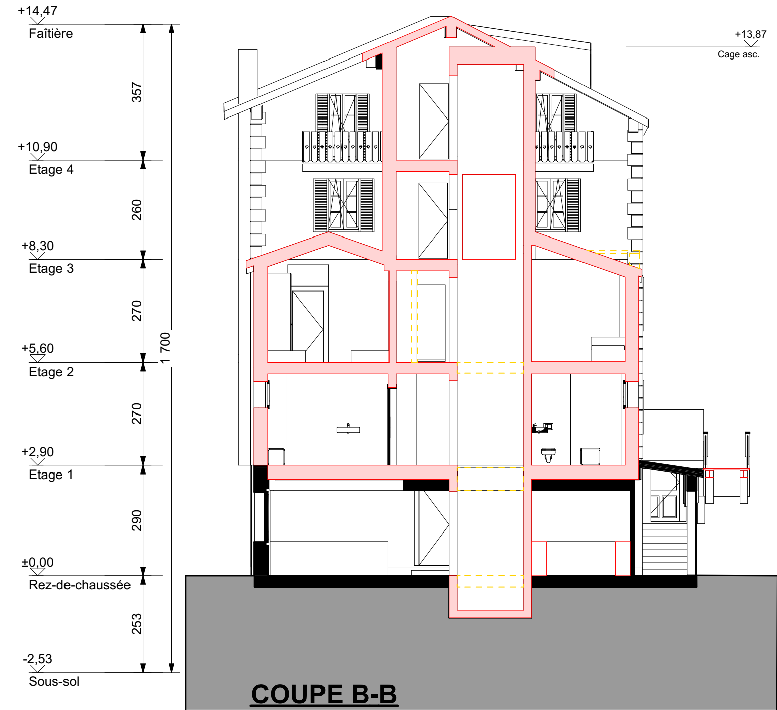
COUPE B-B
